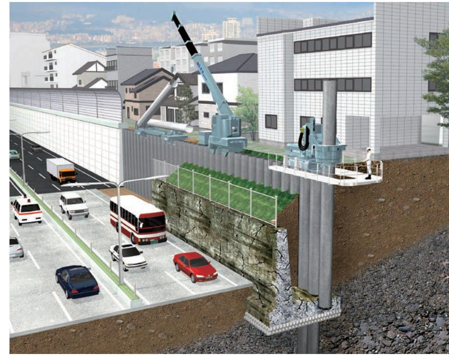
適用例 加世田道路拡幅擁壁建設工事
